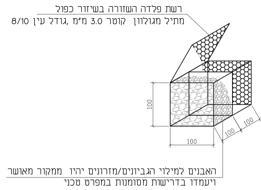
פרט גביונים 1 : 25
