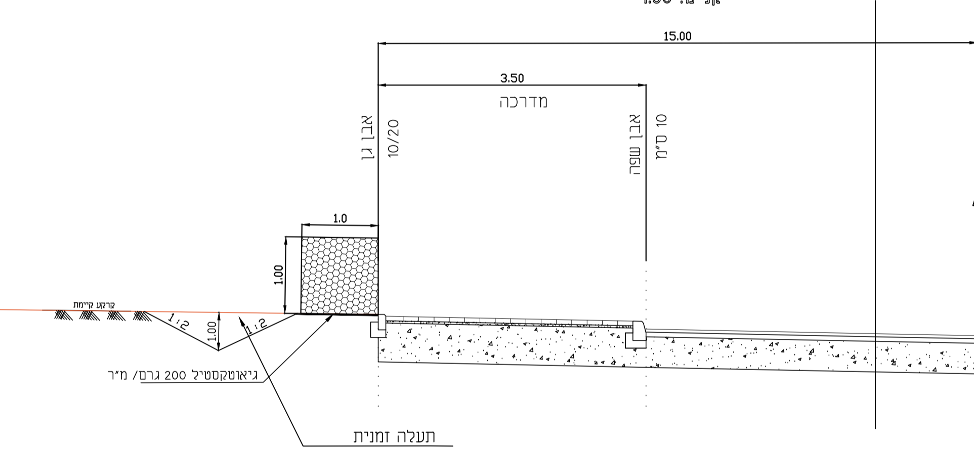
חתך אי - אי קני"ם: 1:50
